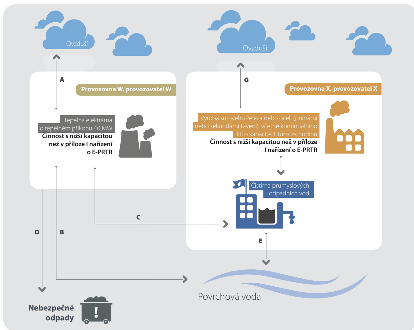
Obrázek 2: Průmyslový komplex se dvěma provozovnami s činností s nižší kapacitou než v příloze I nařízení o E-PRTR
