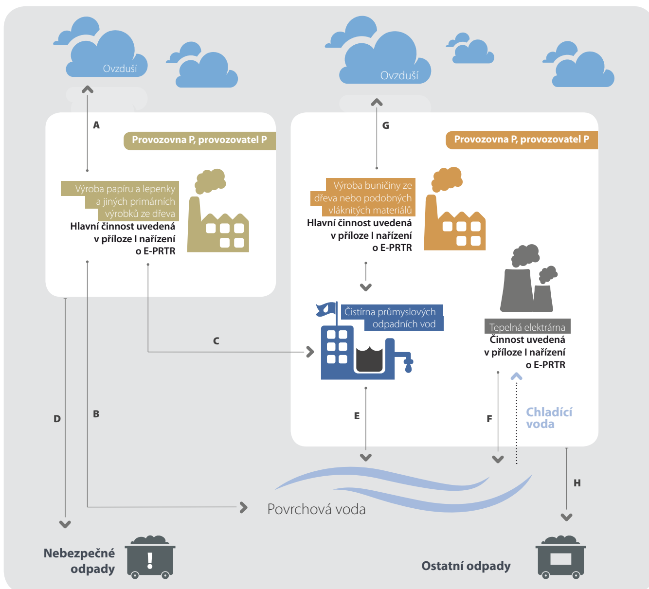
Obrázek 1: Průmyslový komplex se dvěma provozovami s činnostmi podle přílohy I nařízení o E-PRTR
